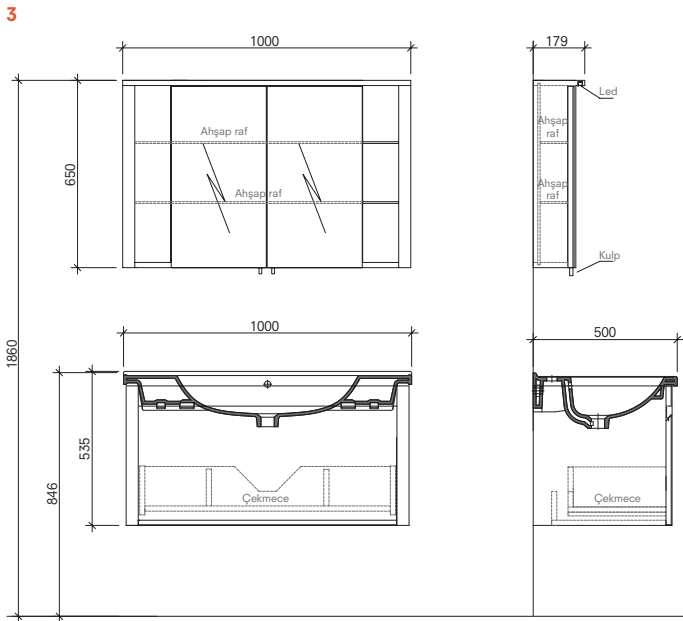
100 cm Set Ön ve Yan Görünüş
