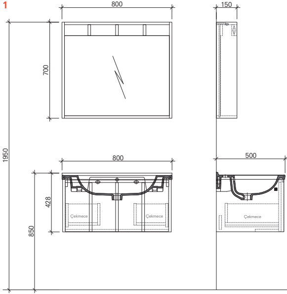
80 cm Set Ön ve Yan Görünüş
