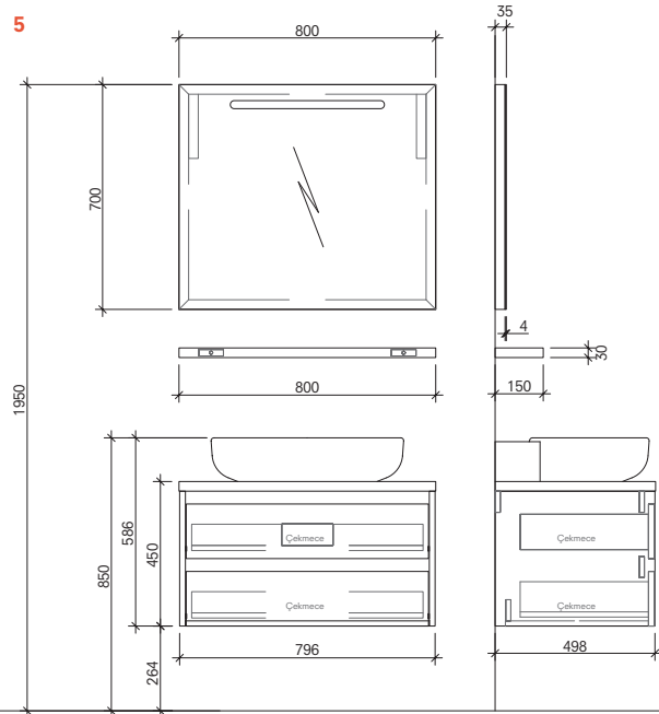
80 cm Set Ön ve Yan Görünüş (Aydınlatmalı ayna + Etajer)
