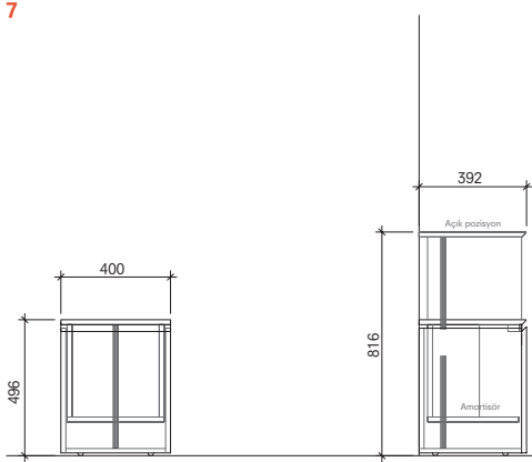
Amortisörlü Yer Modülü 40 cm Ön ve Yan Görünüş
