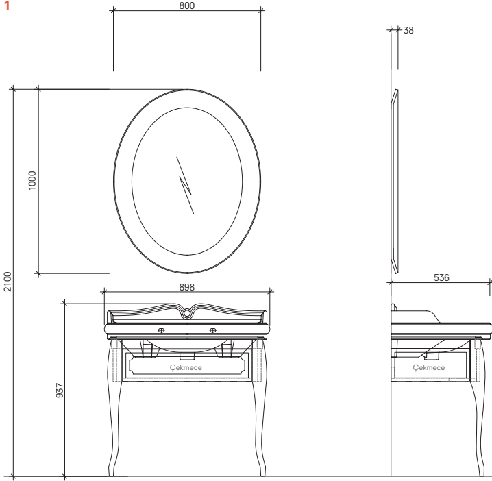
90 cm Set Ön ve Yan Görünüş
