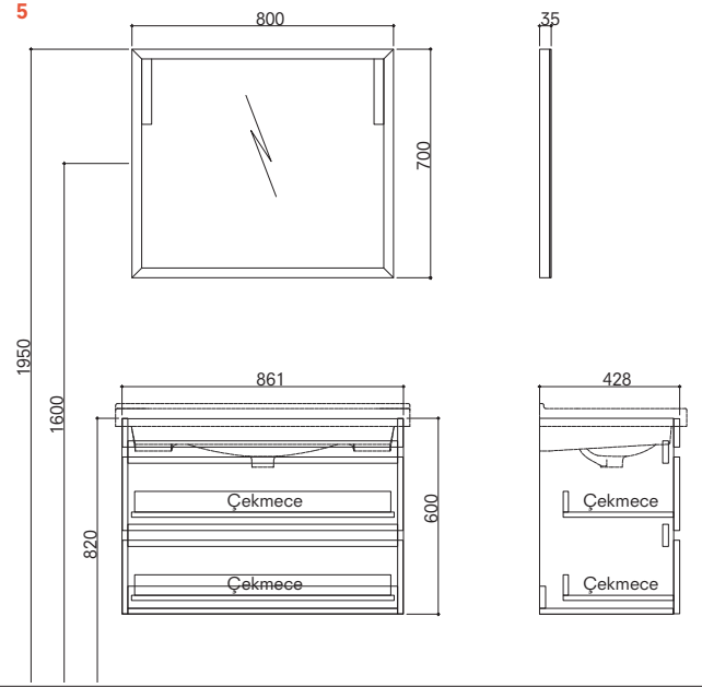
90 cm Set Çekmeceli Ön ve Yan Görünüş (Düz Ayna)
