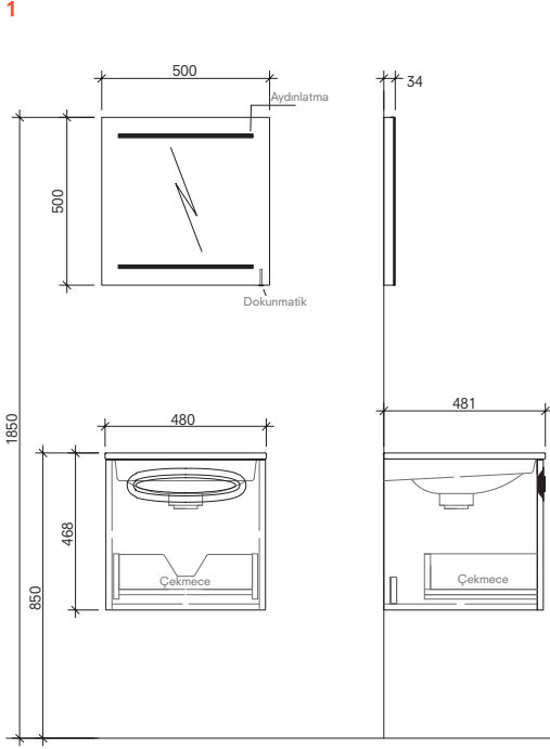
48 cm Set (Etajerli) Ön ve Yan Görünüş
