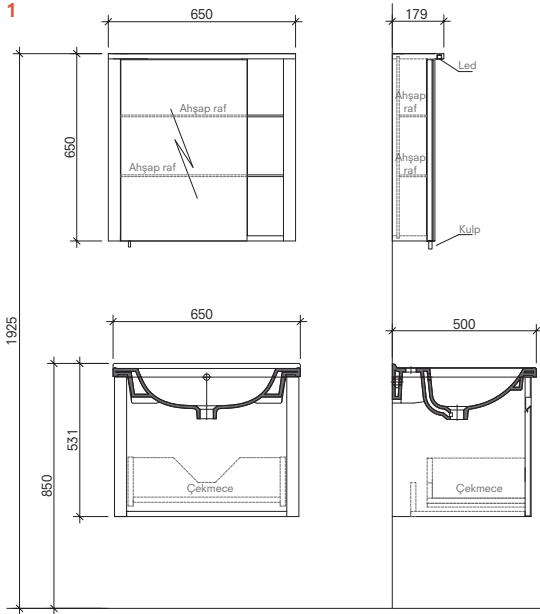
65 cm Set Ön ve Yan Görünüş
