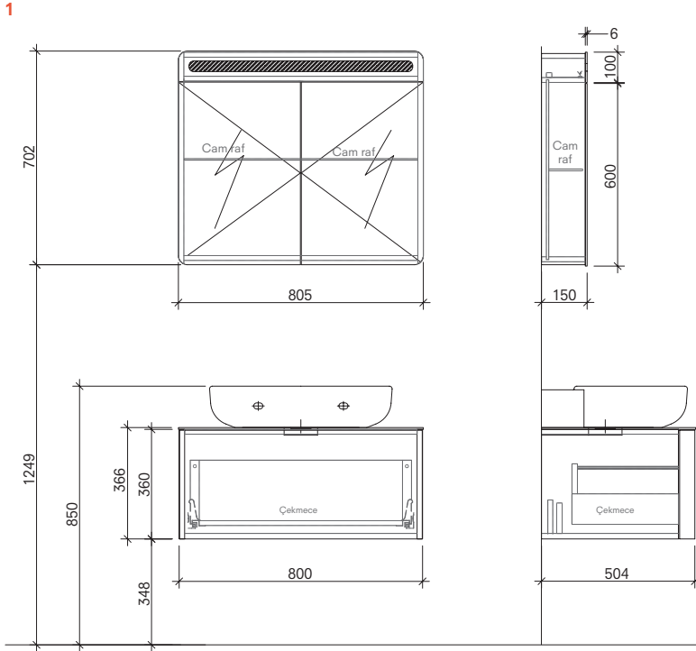
80 cm Set Ön ve Yan Görünüş
