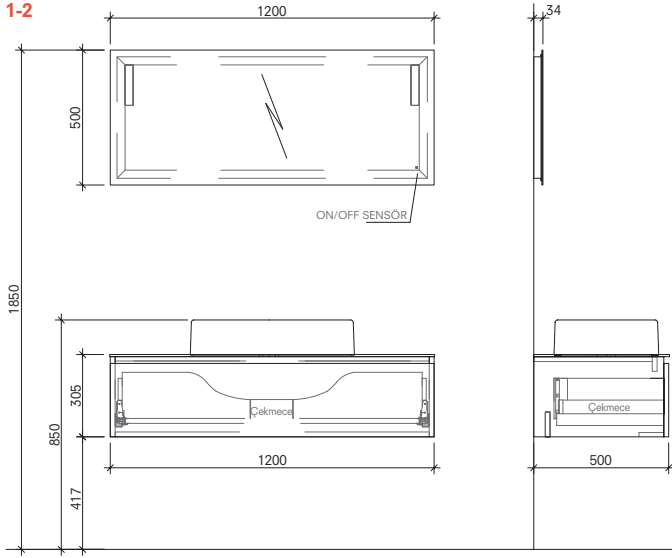
120 cm Set Ön ve Yan Görünüş
