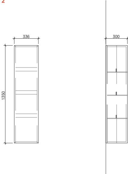
Boy Dolabı 35 cm Ön ve Yan Görünüş
