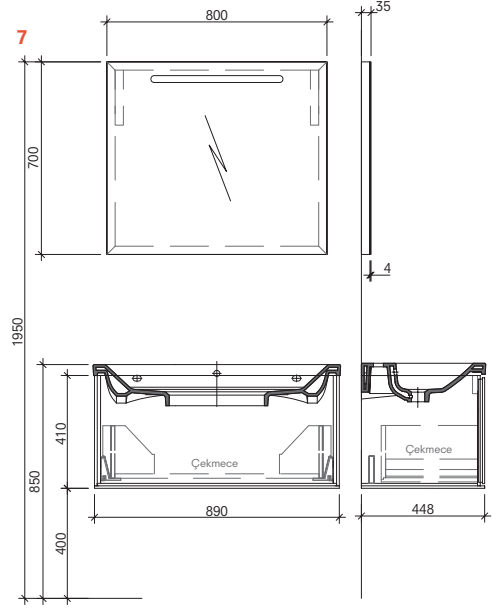
90 cm Set (Etajerli) Ön ve Yan Görünüş
