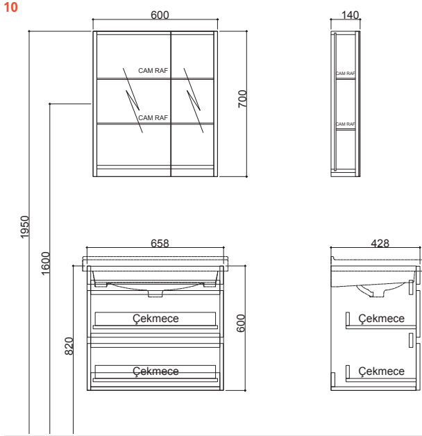
70 cm Set Çekmeceli Ön ve Yan Görünüş (Ayna Dolabı (Aydınlatmasız))
