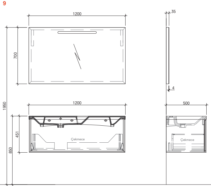
120 cm Set (Sağ Etajerli) Ön ve Yan Görünüş
