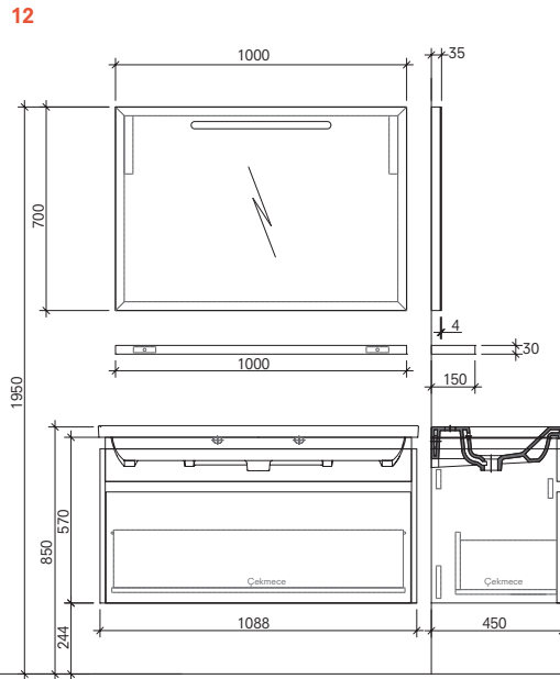
110 cm Set Ön ve Yan Görünüş (Aydınlatmalı ayna +Etajer)
