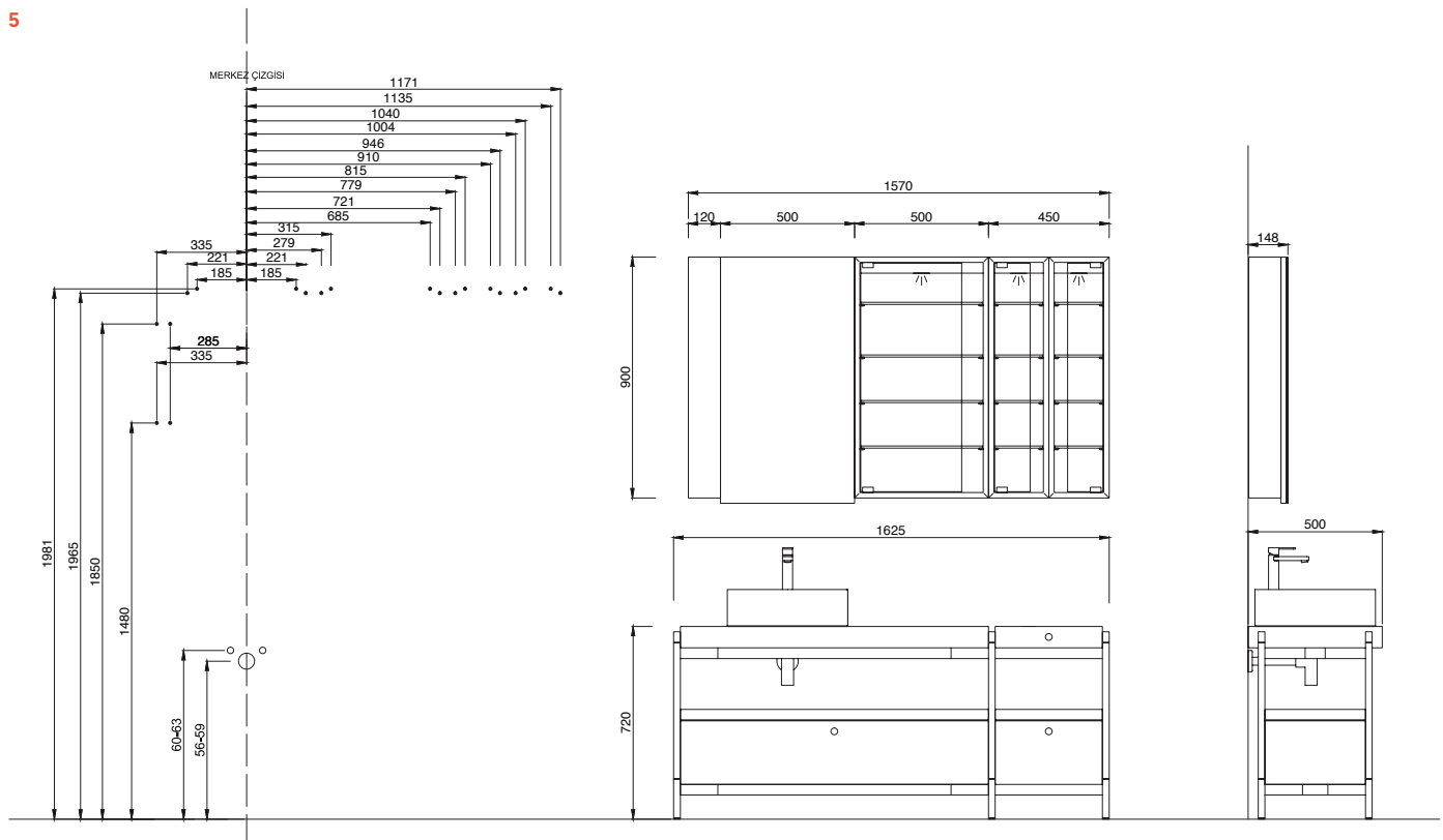
165 cm Set Ön, Yan Görünüş ve Montaj Delik Ölçüleri
