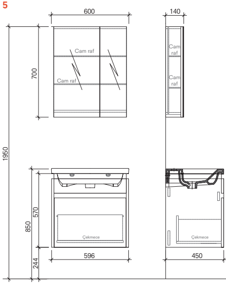
60 cm Set Ön ve Yan Görünüş (Ayna Dolabı (Aydınlatmasız))
