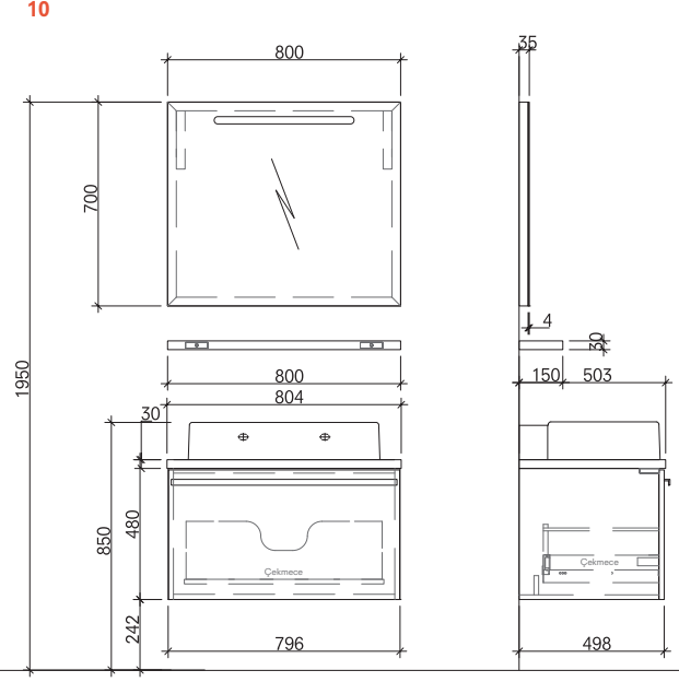
80 cm Set Derin Ön ve Yan Görünüş
