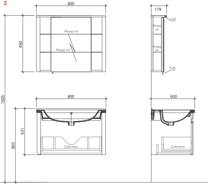
80 cm Set Ön ve Yan Görünüş
