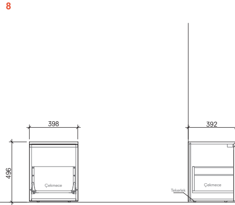
Tekerlekli Yer Modülü 40 cm Ön ve Yan Görünüş
