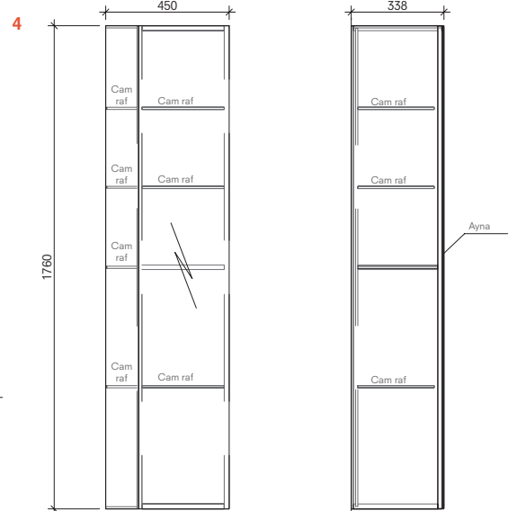
45 cm Boy Dolap Sol Ön ve Yan Görünüş
