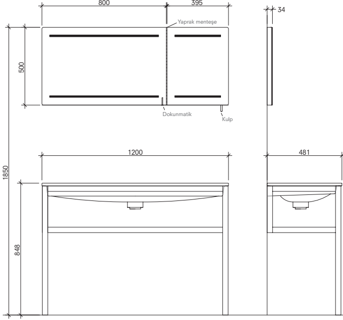
120 cm Set Çanak Lavabolu (Sol) Ön ve Yan Görünüş
