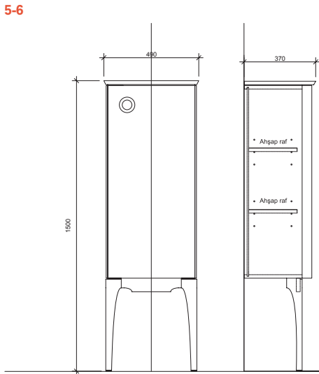
50 cm Boy Dolap Ön ve Yan Görünüş
