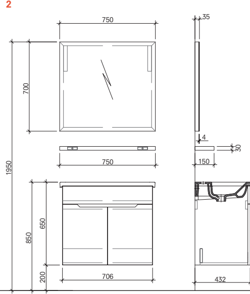
75 cm Set Ön ve Yan Görünüş
