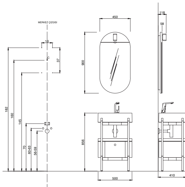
Elips Set Ön, Yan Görünüş ve Montaj Delik Ölçüleri
