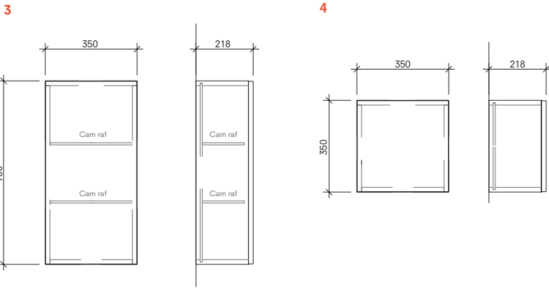
Yer Modülü Puf 35 cm Ön ve Yan Görünüş
