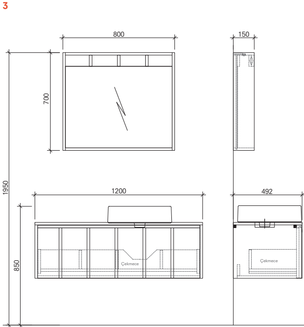
120 cm Set (80 cm Ayna Dolabı) Ön ve Yan Görünüş
