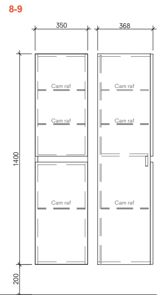
Boy Dolap 35 cm Ön ve Yan Görünüş
