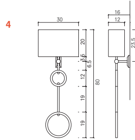
Kumaş Aplik Ön ve Yan Görünüş (Havluluk Aksesuar ile Birlikte)
