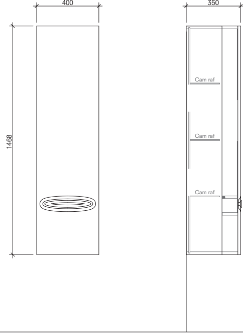
Boy Dolap 40 cm (Sol-Sağ) Ön ve Yan Görünüş
