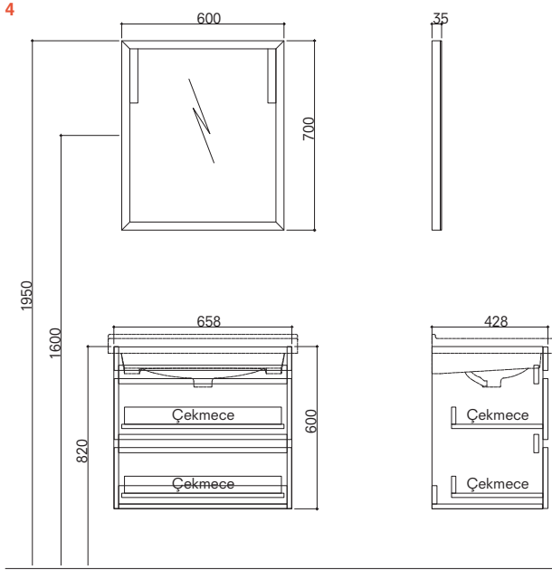
70 cm Set Çekmeceli Ön ve Yan Görünüş (Düz Ayna)
