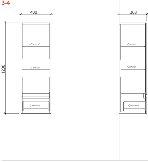
Alt Dolap 40 cm Ön ve Yan Görünüş
