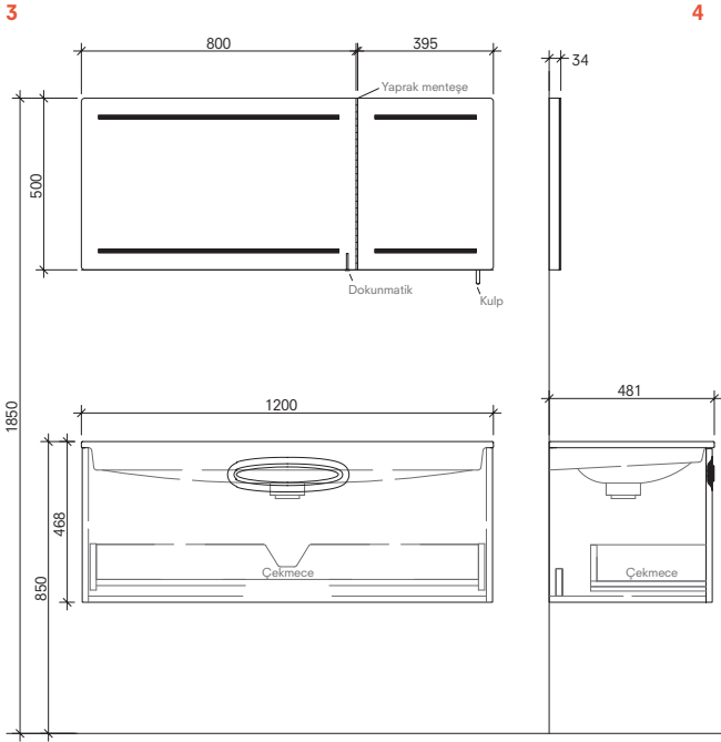
120 cm Set (Etajerli) Ön ve Yan Görünüş
