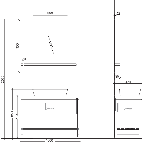
100 cm Set Ön ve Yan Görünüş
