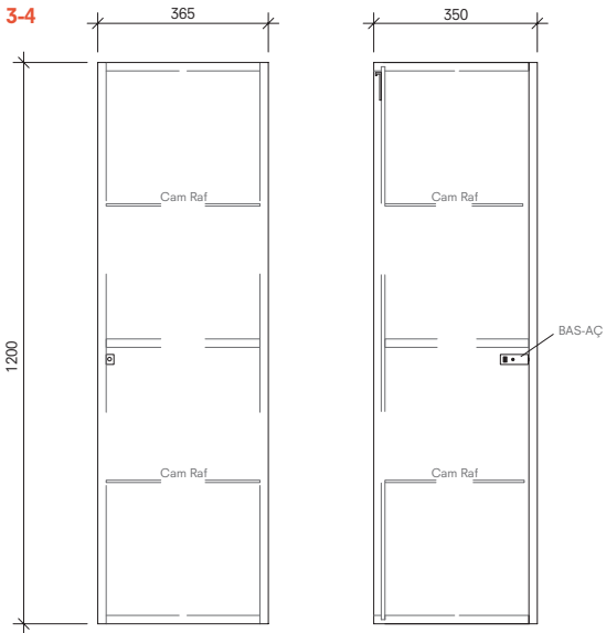
Boy Dolabı 35 cm Ön ve Yan Görünüş
