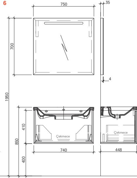
75 cm Set (Etajerli) Ön ve Yan Görünüş
