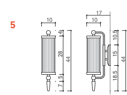
Cam Aplik Ön ve Yan Görünüş
