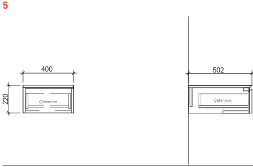
Amortisörlü Yer Modülü 40 cm Ön ve Yan Görünüş
