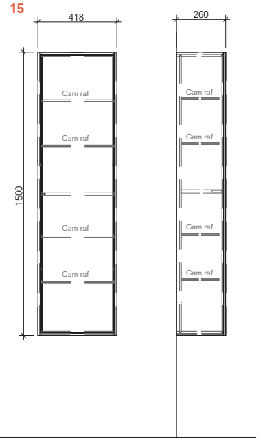
Boy Dolap 150 cm Sağ/Sol Ön ve Yan Görünüş
