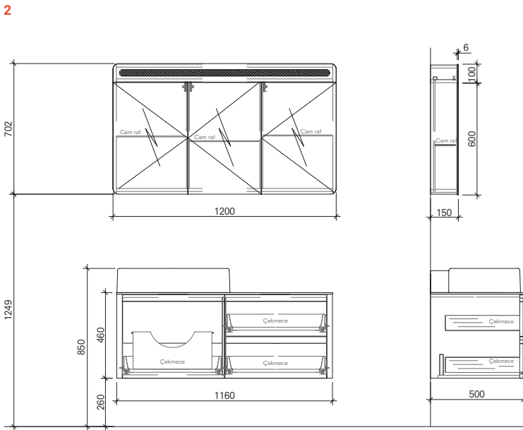
120 cm Set Ön ve Yan Görünüş
