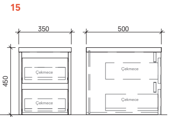
Asma Dolap 35 cm Ön ve Yan Görünüş
