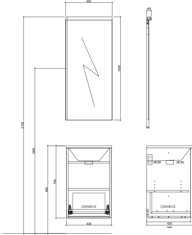
Cam Rafı Yan Alt Modül 40 cm Ön ve Yan Görünüş
