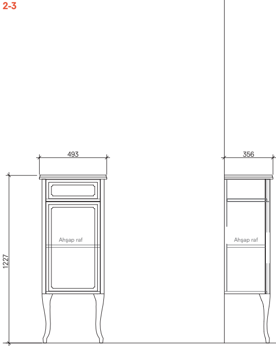
Boy Dolap 50 cm Sağ/Sol Ön ve Yan Görünüş
