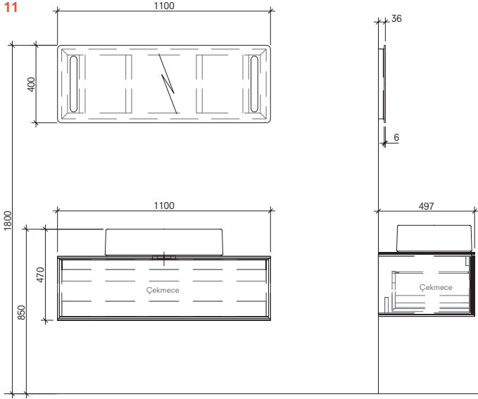
110 cm set (Dikdörtgen Çanak Lavabolu) Ön ve Yan Görünüş
