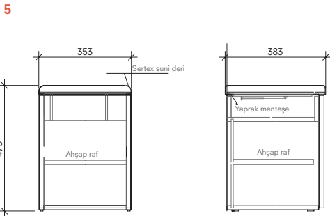
Yer Modülü Puf 35 cm Ön ve Yan Görünüş
