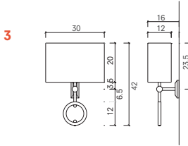
Kumaş Aplik Ön ve Yan Görünüş
