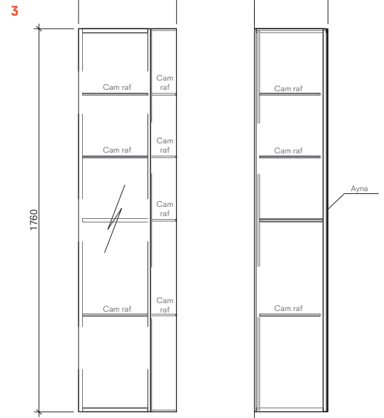
45 cm Boy Dolap Sağ Ön ve Yan Görünüş
