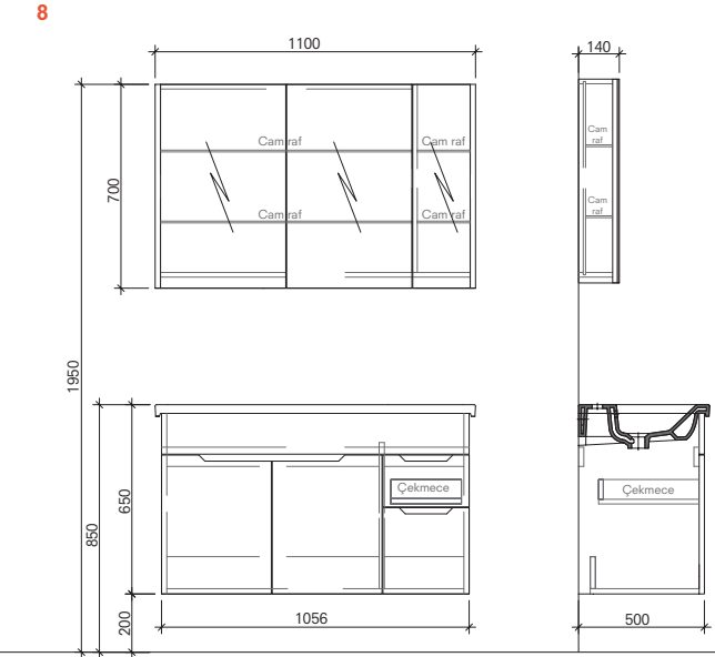
110 cm Set Ön ve Yan Görünüş
