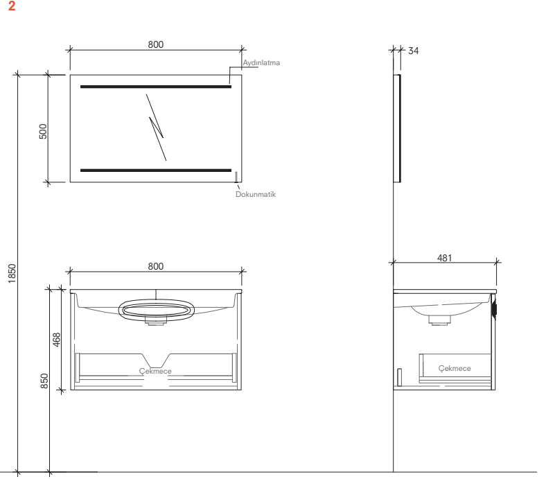
80 cm Set (Etajerli) Ön ve Yan Görünüş
