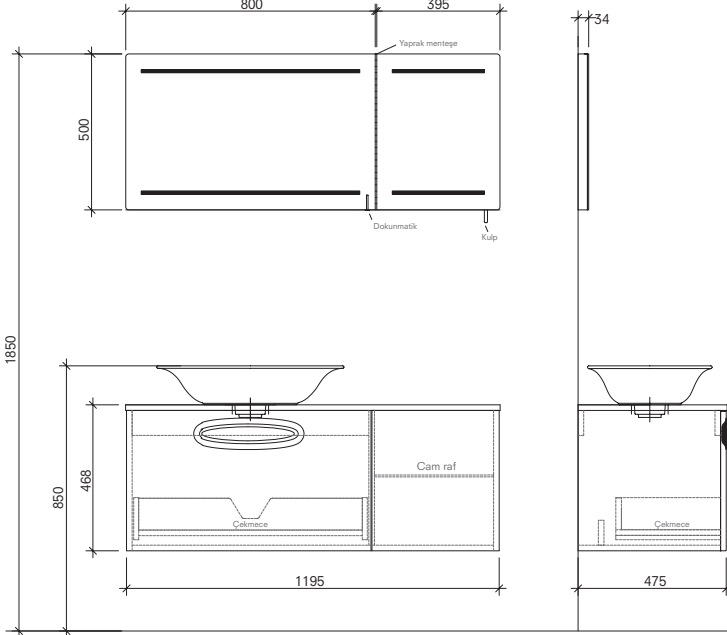
120 cm Set Çanak Lavabolu (Sol) Ön ve Yan Görünüş
