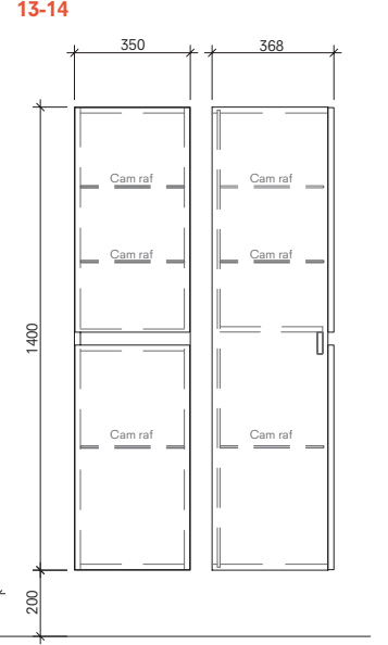
Boy Dolap 35 cm Ön ve Yan Görünüş
