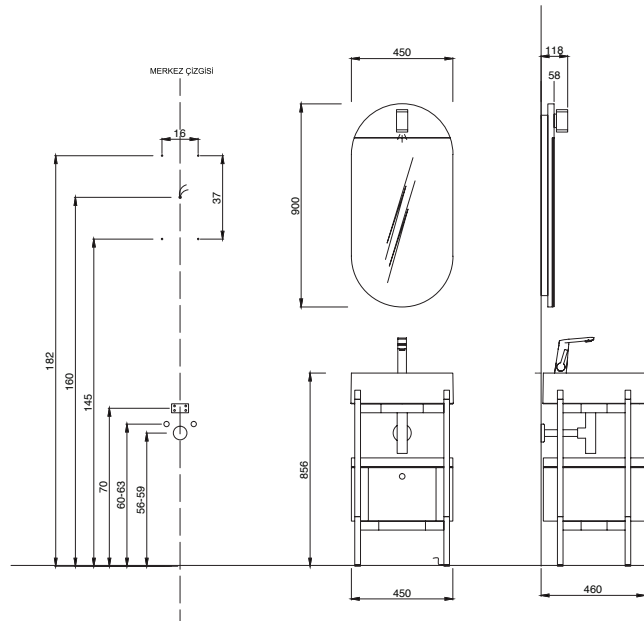
Yuvarlak Set Ön, Yan Görünüş ve Montaj Delik Ölçüleri
